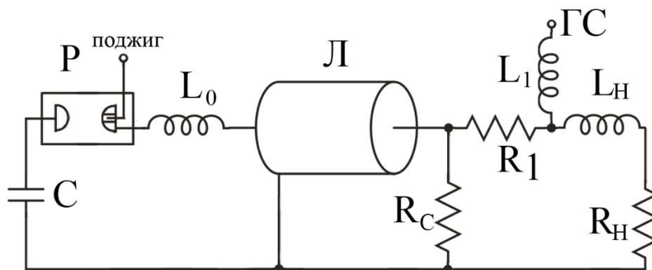
Рис. 1 Схема электроразрядного контура установки: C – емкость конденсаторной батареи, P – разрядник, L_0 – индуктивность внешней цепи, R_1 \sim 0,5 \text{ Ом} – дополнительный резистор, L – кабельная линия, L_H, R_H – индуктивность и омическое сопротивление проволоочки, R_c \sim 9 \text{ Ом} – согласующий резистор.
